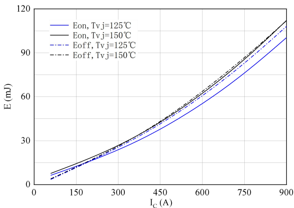
图 5. 开关损耗 逆变器
